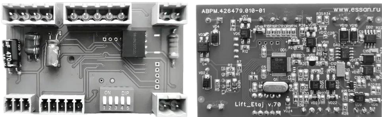
Рис. 12 Этажный контроллер. Передняя и задняя сторона без корпуса.
