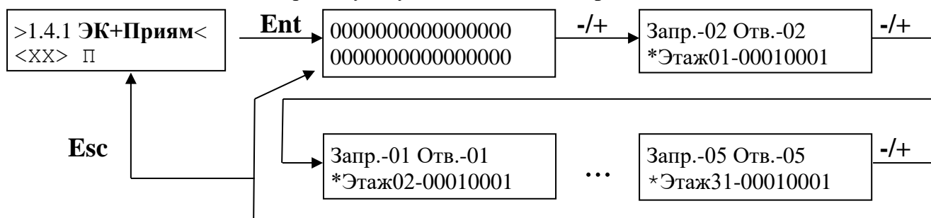
Рис. 30 Структура подменю >1.4 Этажи
