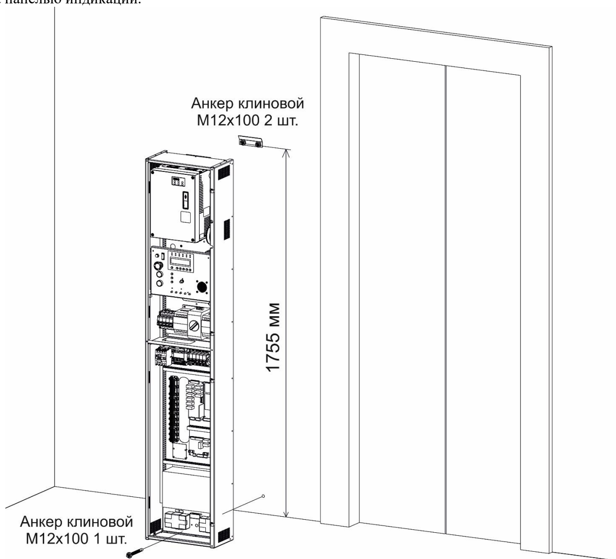
Рис. 19. Схема установки СУЛ СОЮЗ 2М-БМ на стену
