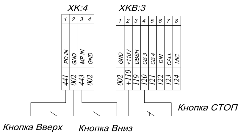
Рис. 48 Подключение поста ревизии.
