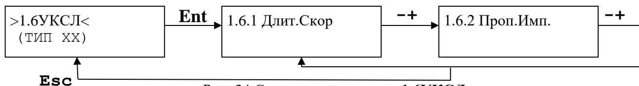
Рис. 34 Структура подменю >1.6УКСЛ<
