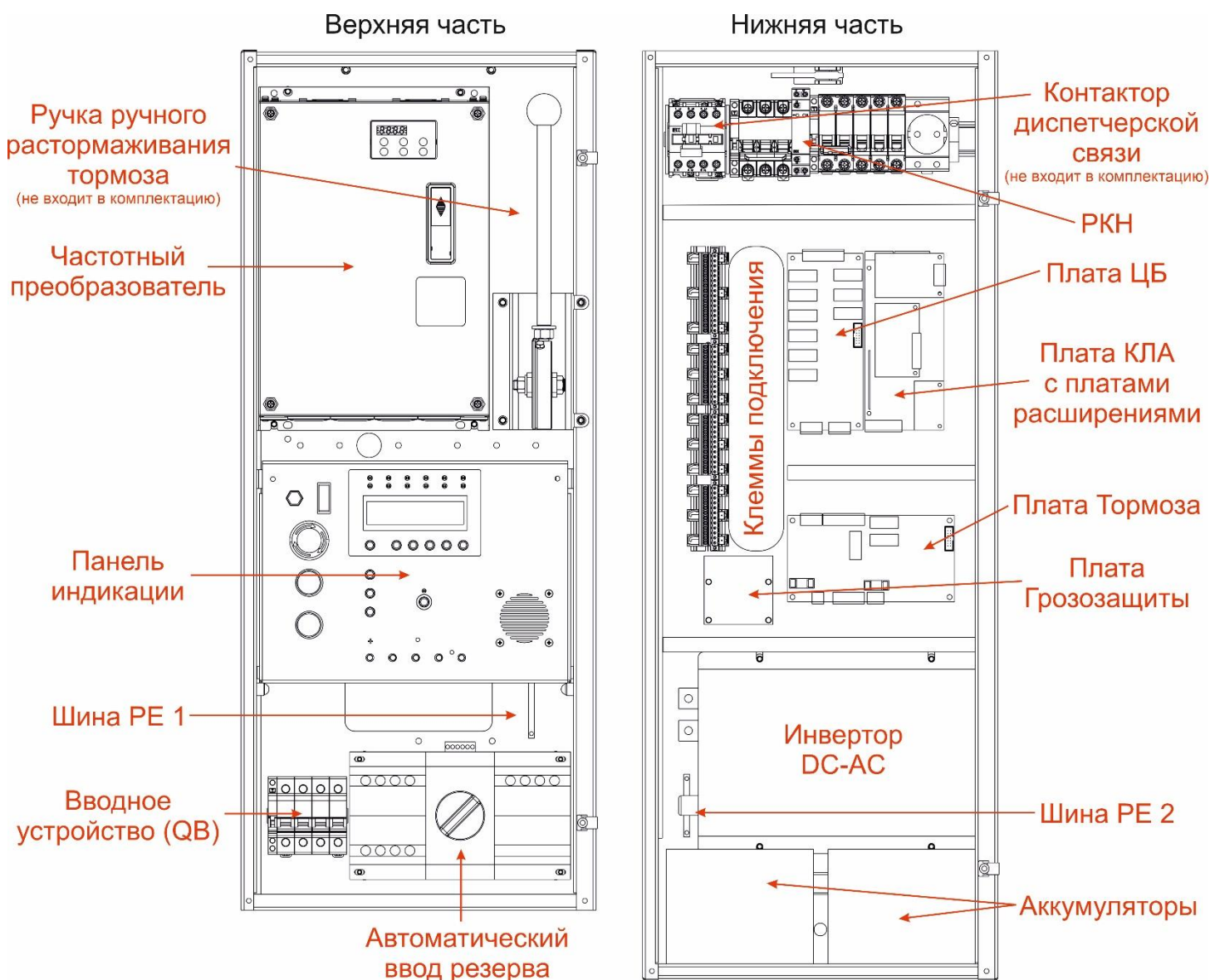
Рис. 18 Внешний вид станции управления СОЮЗ 2М-БМ
