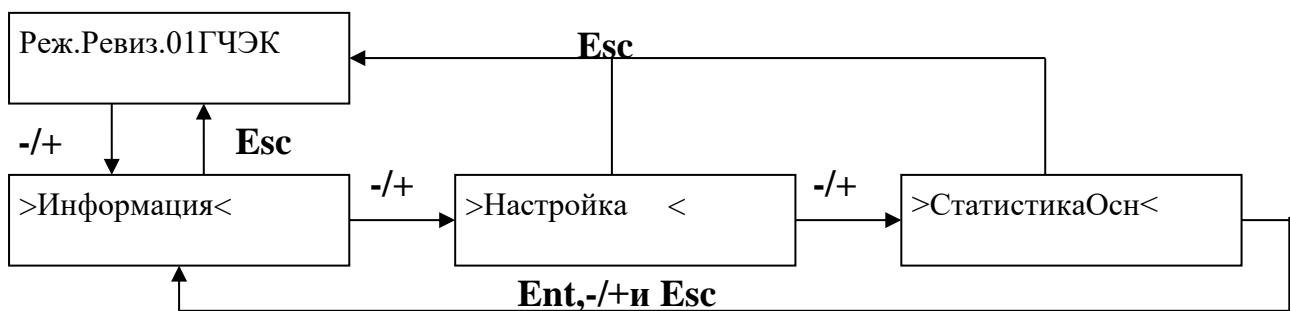
Рис. 25 Структура меню в режиме «РЕВИЗИЯ»
