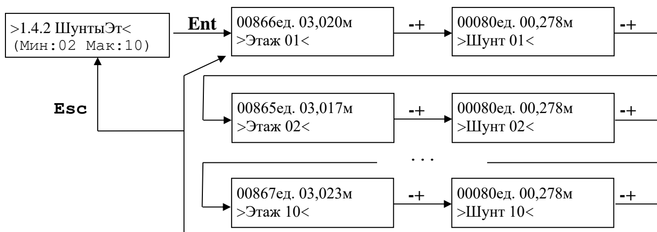
Рис. 31 Структура подменю >1.4.2 ШунтыЭт<
