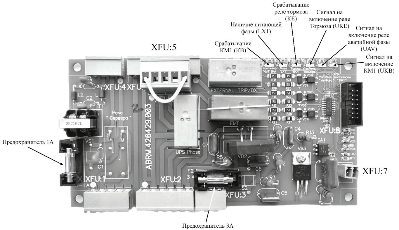
Рис. 6 Плата Филтр УК
