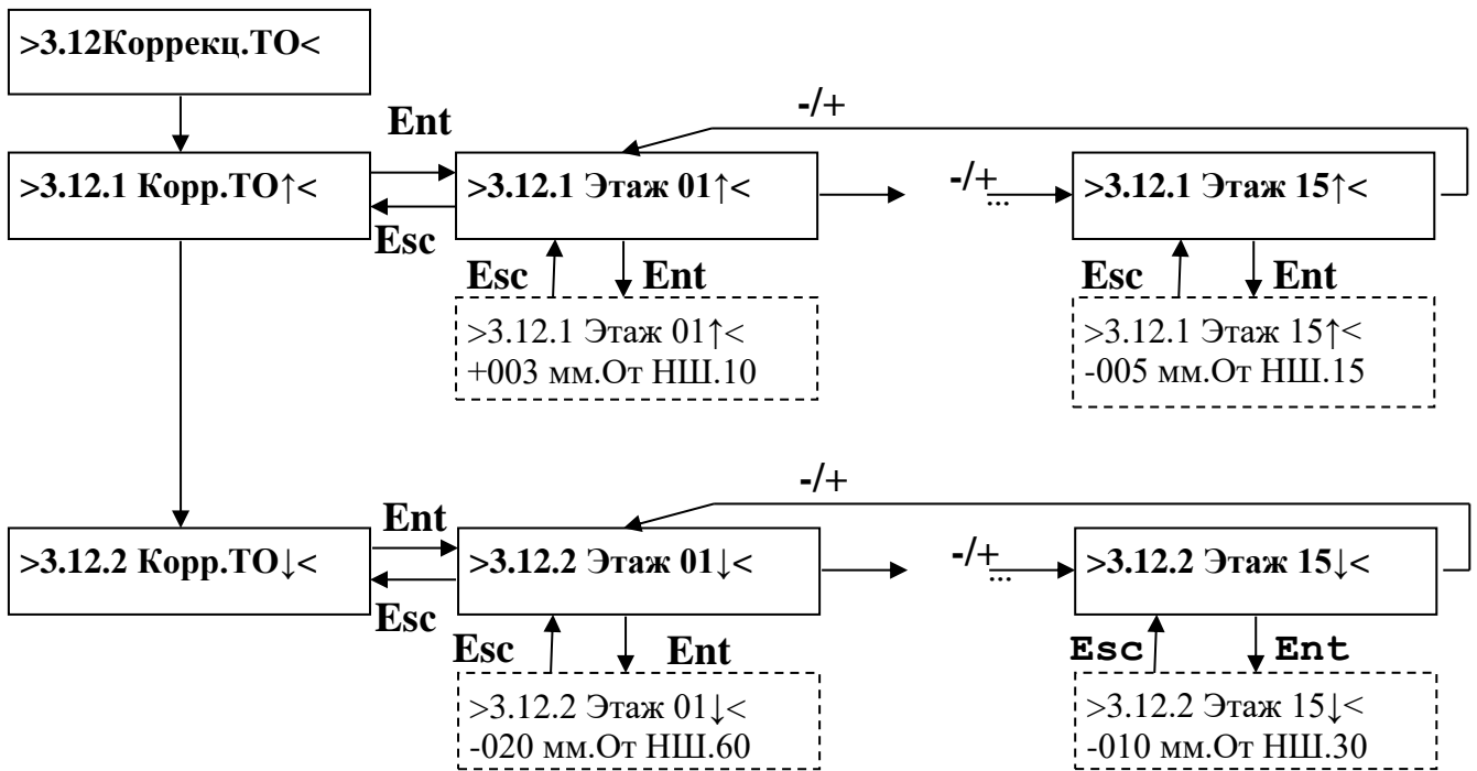
Рис. 47 Структура подменю >3.12Коррекц.ТО<
