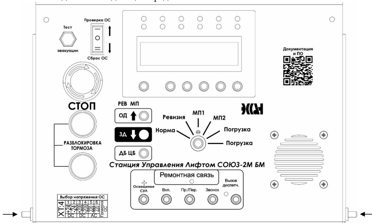
Рис. 20 Панель индикации СУЛ СОЮЗ 2М-БМ
