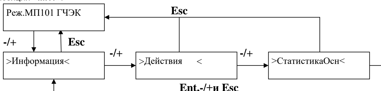
Рис. 26 Структура меню в режиме «МП1».
