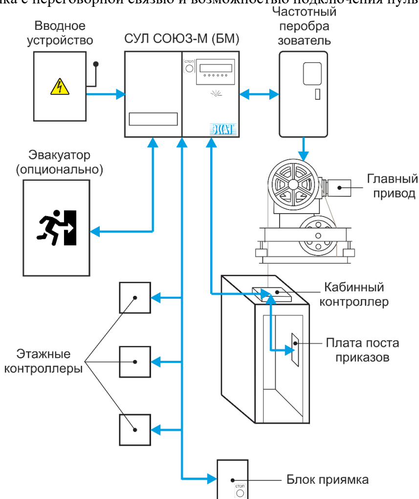
Рис. 1 Структурная схема СУЛ.
