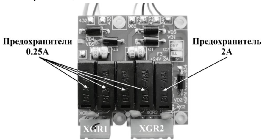
Рис. 11 Плата грозозащиты
