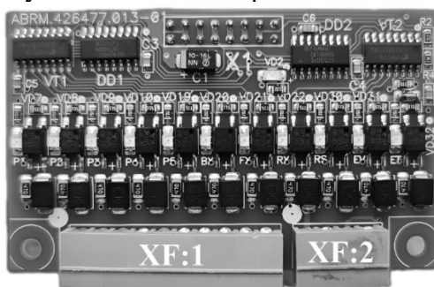
Рис. 10 Плата ЧП-KEY
