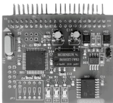
Рис. 9 Плата модуля групповой работы
