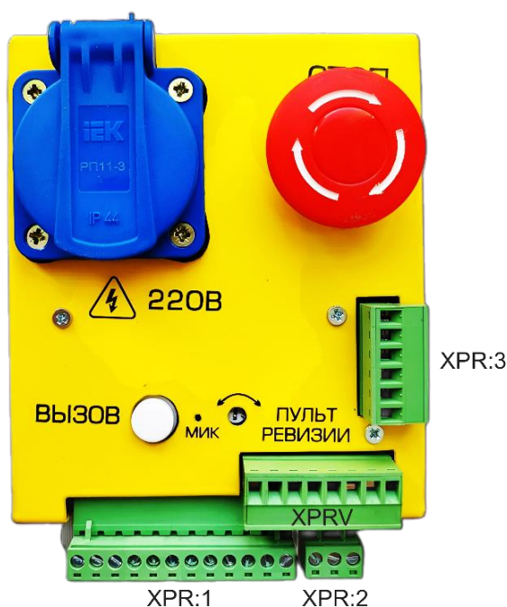
Рис. 15 Блок прямка
