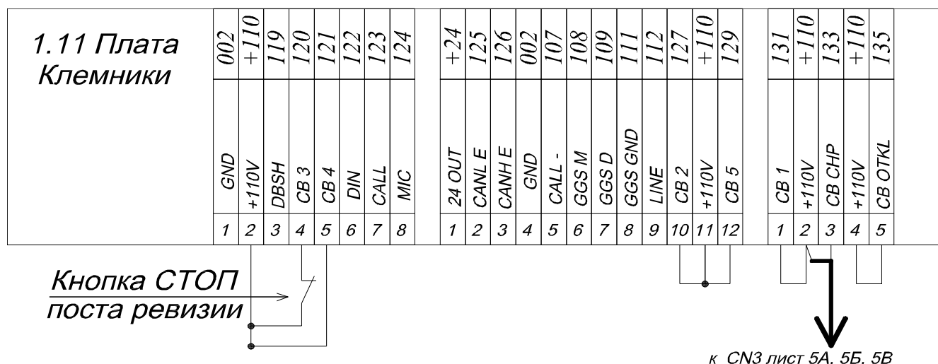
Рис. 4б Подключение перемычек.
