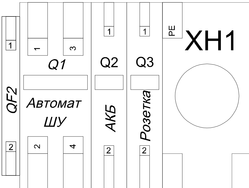
Рис. 3б Силовые автоматы в шкафу управления «Союз БМ».
